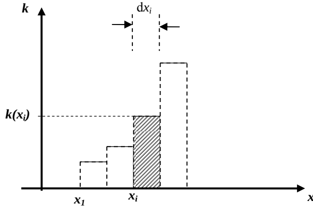
Figura 5. Representación, en el sistema de coordenadas k - x , del intento de mejora de la estimación del \Delta y mediante el cálculo de dy consecutivas. dy_i = k(x_i) \cdot \Delta x_i es el área del rectángulo rayado. La suma del área de todos los rectángulos es una estimación del \Delta y .
