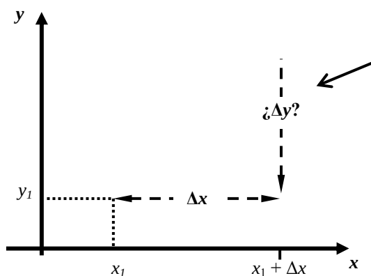
Figura 1. ¿Cuál es el valor de \Delta y correspondiente a ese \Delta x ?
