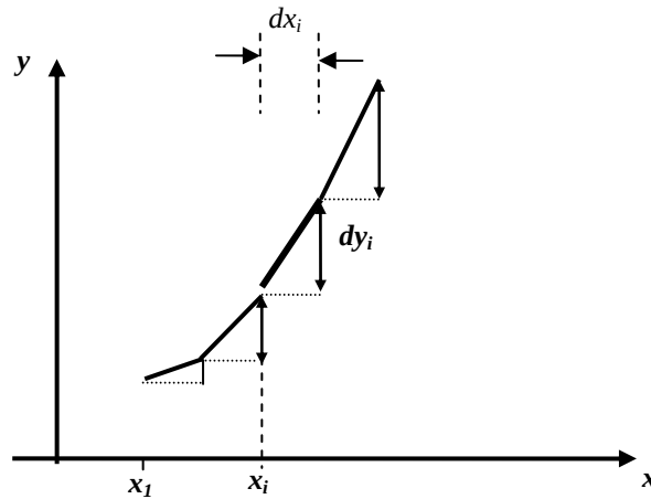
Figura 4. Representación gráfica, en el sistema de coordenadas y - x , del intento de mejora de la estimación del \Delta y mediante el cálculo de dy consecutivas. k(x_i) es la pendiente del segmento más grueso ( dy_i/\Delta x_i ). La suma de todos los segmentos verticales es una estimación del \Delta y .
